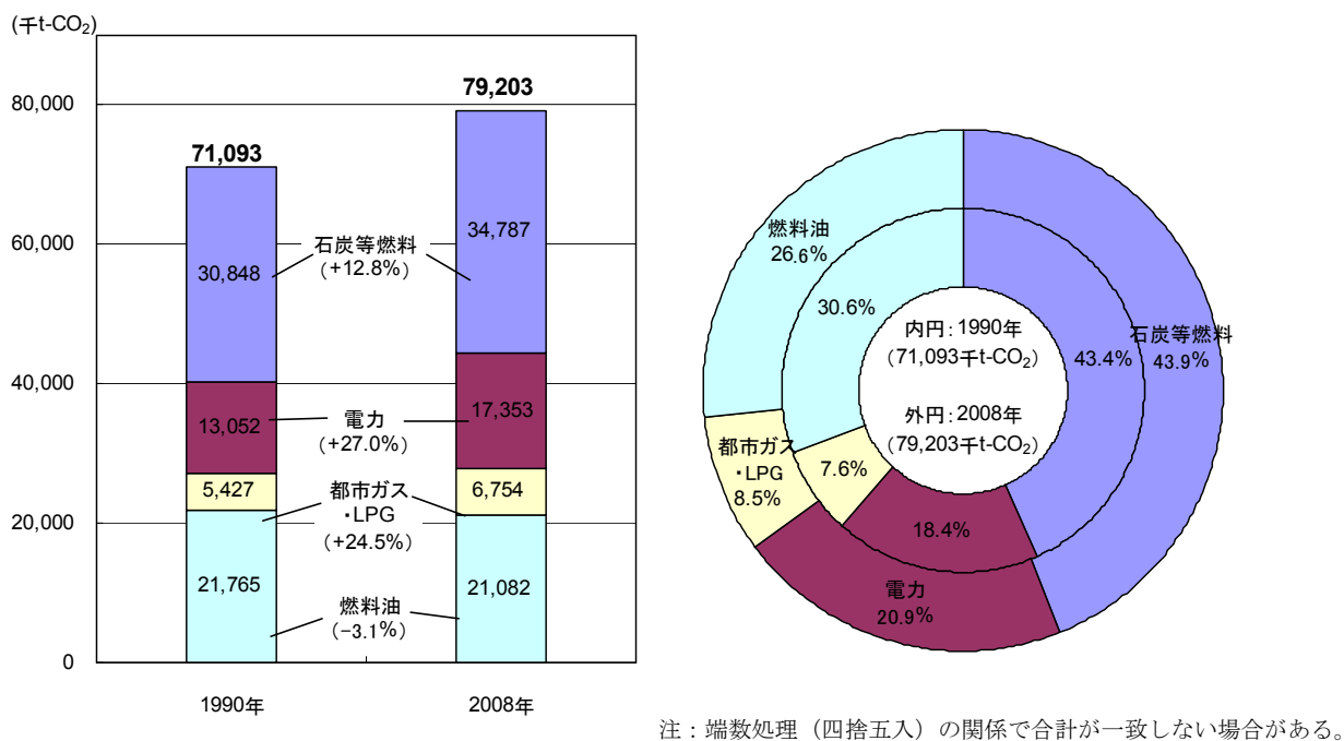
図 1-5 千葉県におけるエネルギー種別二酸化炭素排出量の伸びと構成比
