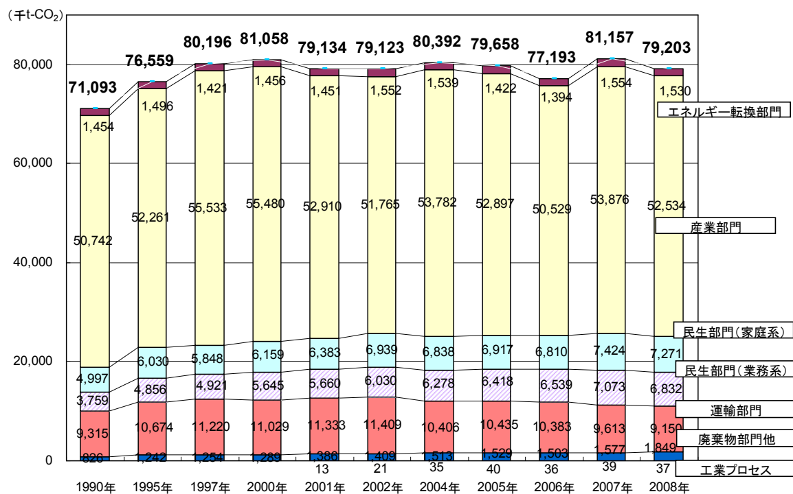
図 1-1 千葉県における二酸化炭素排出量の推移
