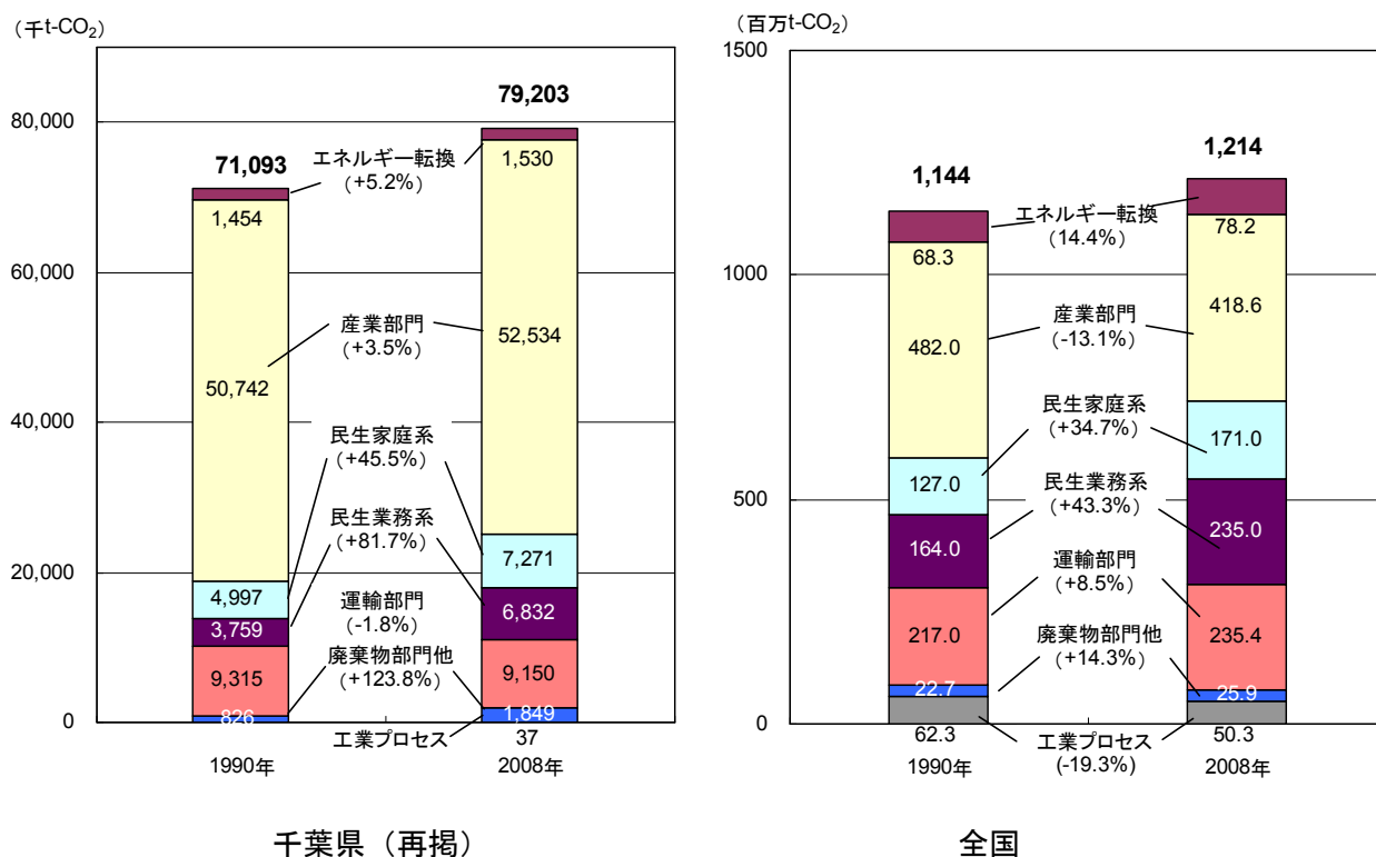
図 1-6 千葉県及び全国の部門別二酸化炭素排出量
