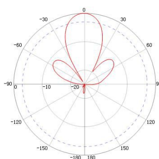
垂直面参考方向图
