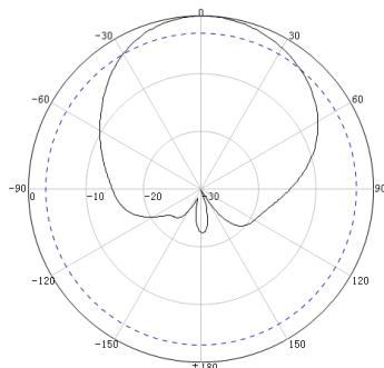
水平面参考方向图
